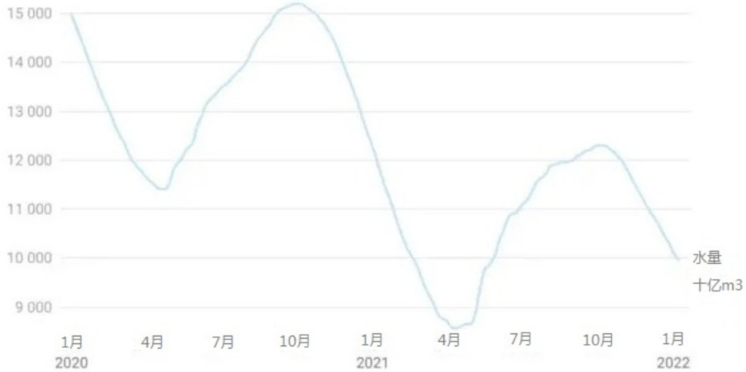
图 1 托克托古尔水库 2020~2022 年水量变化
